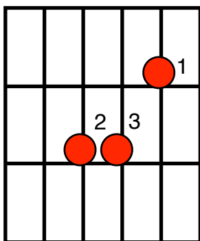
Am [minor]
