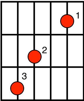
E [major]
