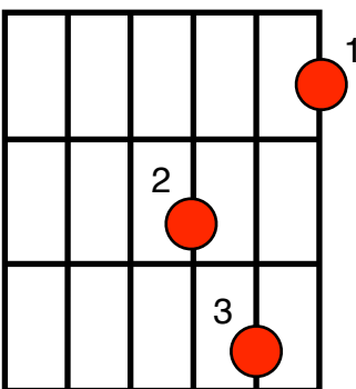
Dm [minor]
