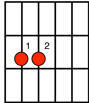
Em [minor]
